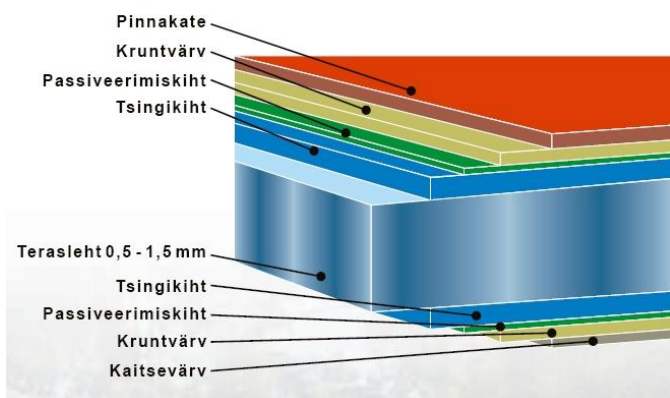
Pinnakattega kuumtsingitud terasplekki ristlõige
